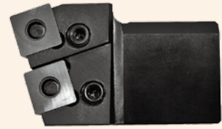
特殊バイトホルダ Special Bite Holder
